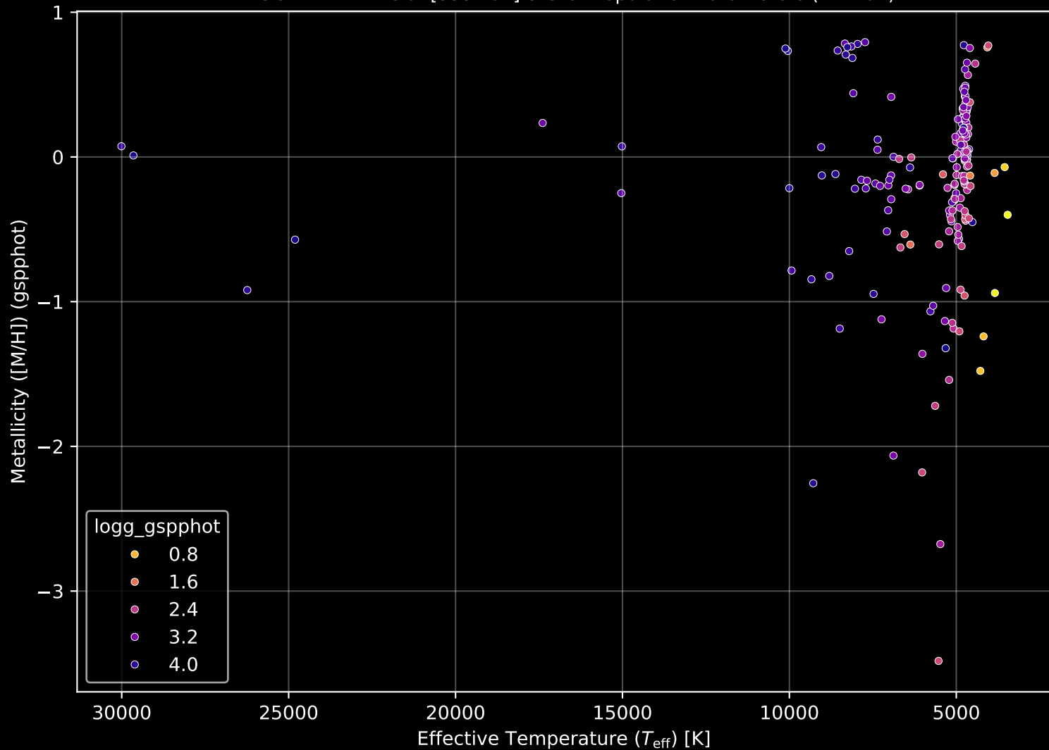
APOGEE DR17 Field: [355+04] Stellar Population Parameters (n= 201)
